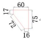
附图2、五边形钢管详细图
